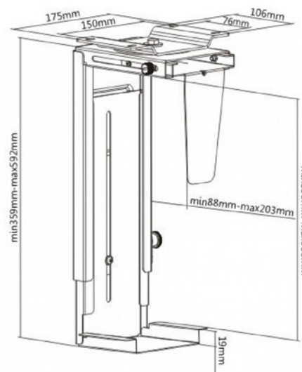
disegno tecnico
